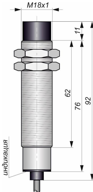
Габаритный чертеж
