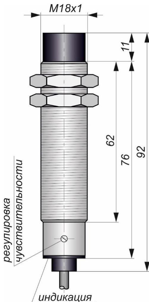
Габаритный чертеж
