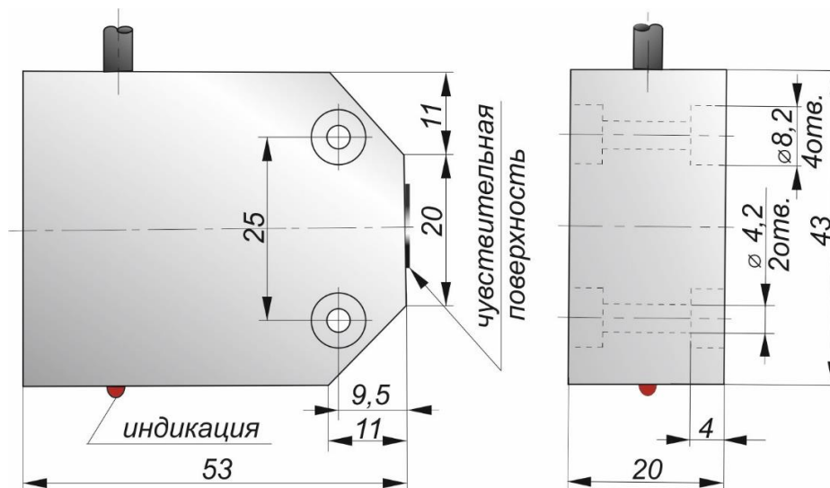
Габаритный чертеж
