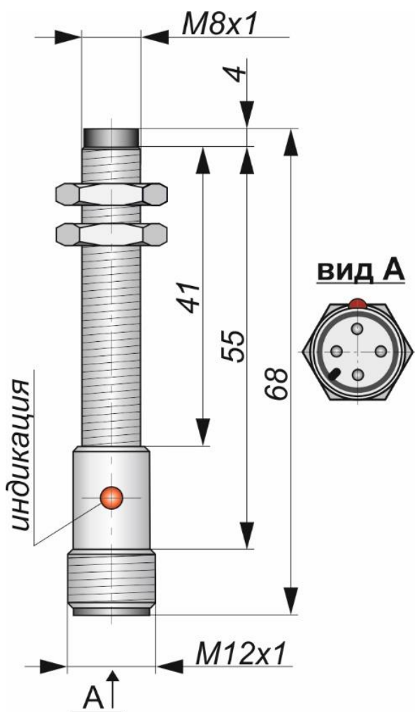
Габаритный чертеж
