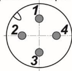
Цоколевка разъема
