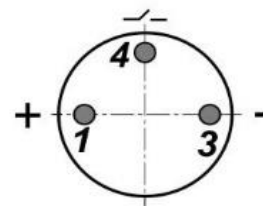
Цоколевка разъема
