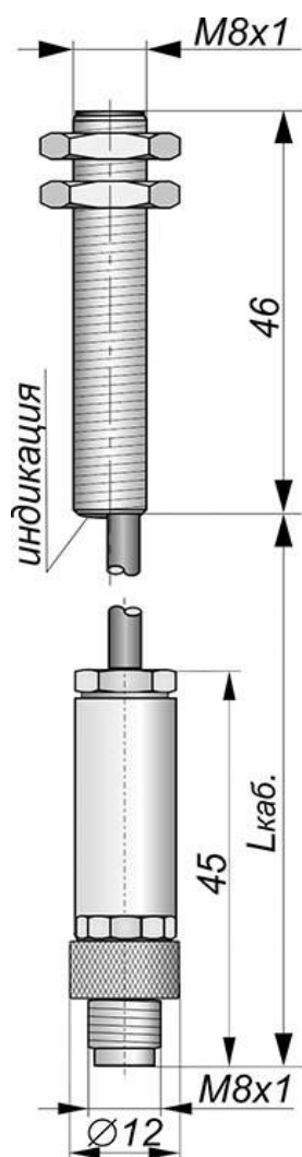
Габаритный чертеж
