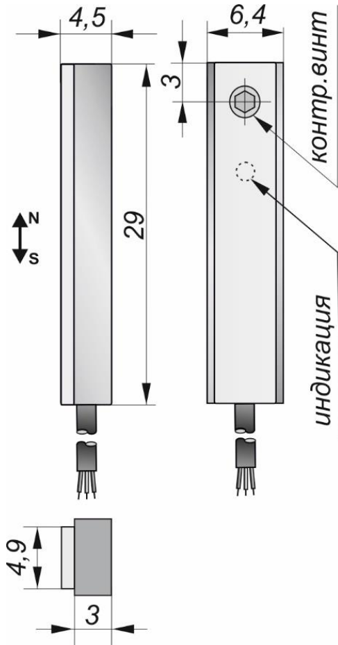
Габаритный чертеж
