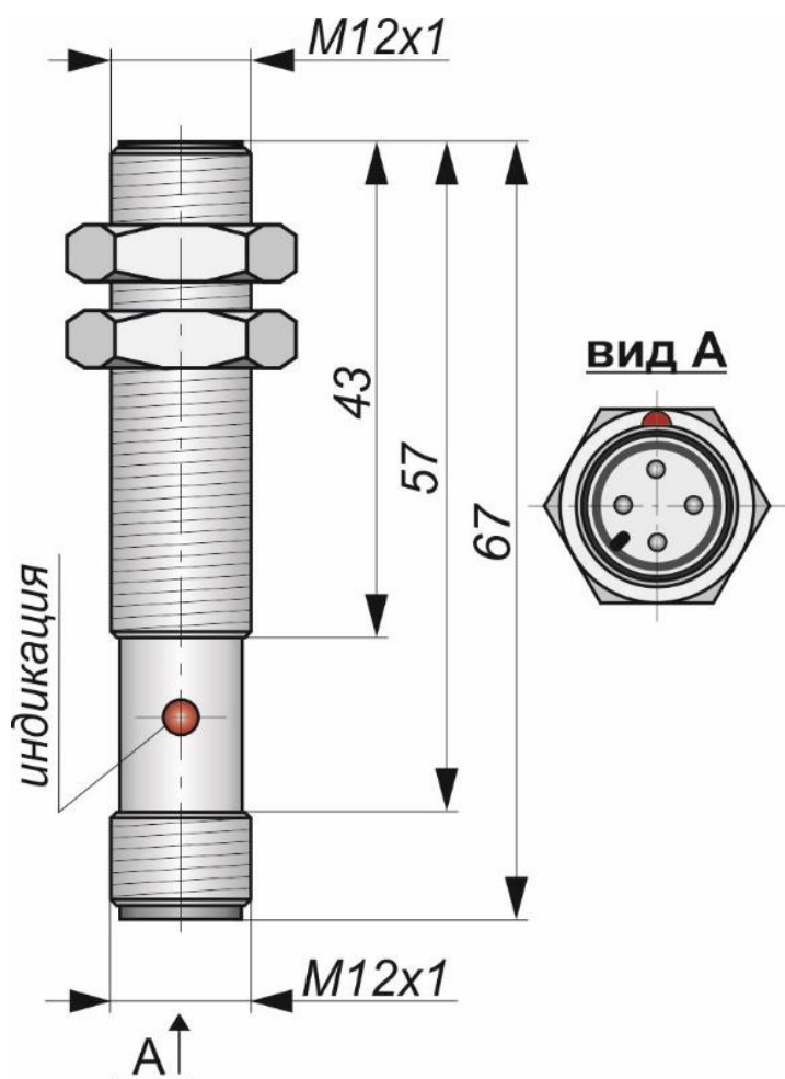
Габаритный чертеж
